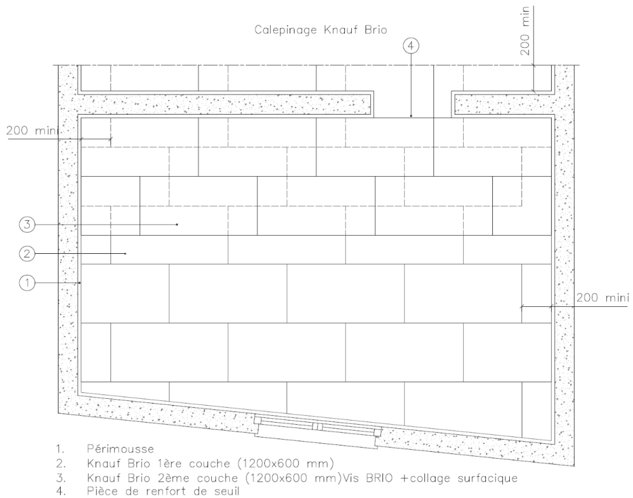
Figure 3 – Calepinage KNAUF BRIO 18
