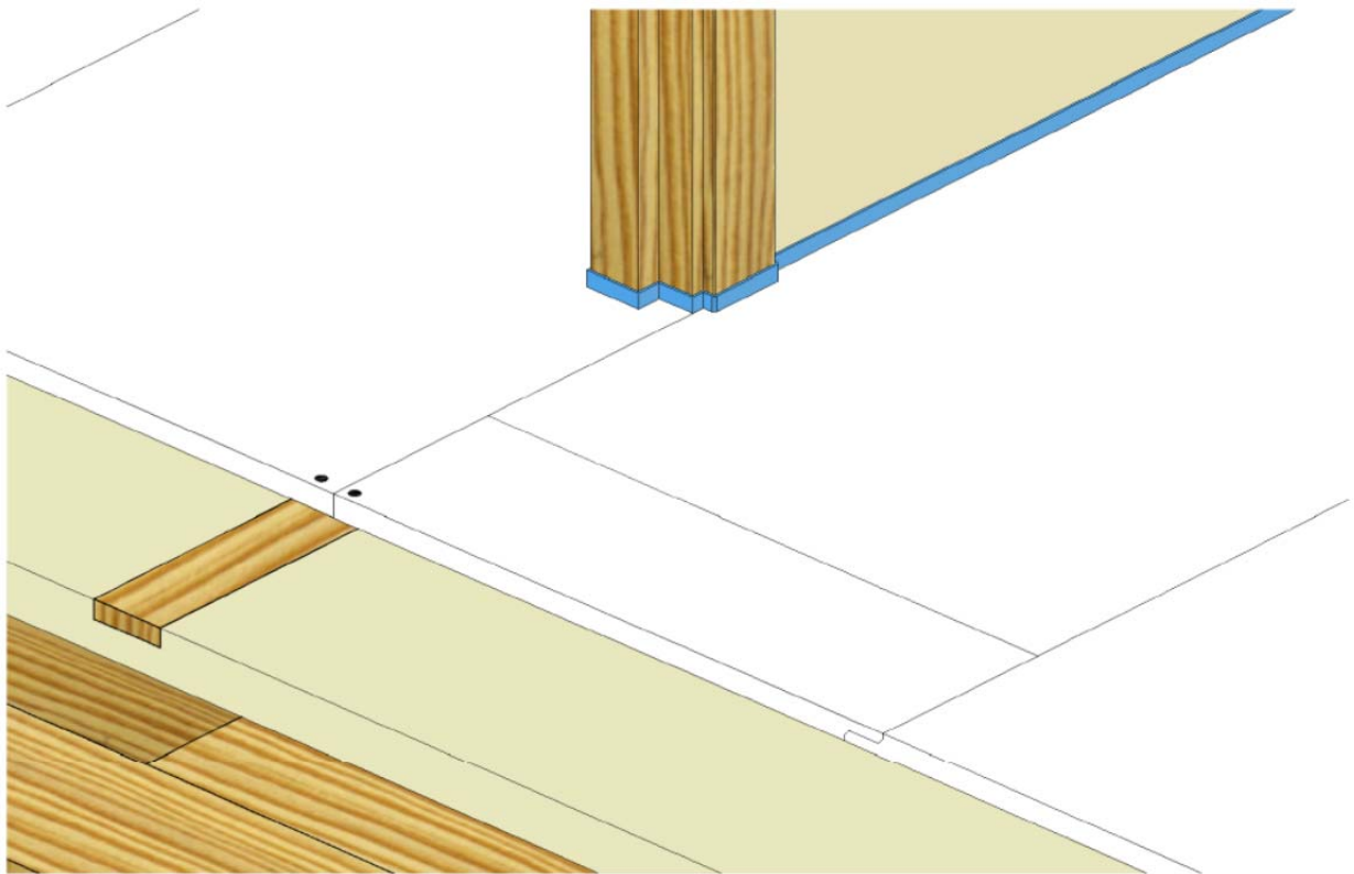
Figure 6 - KNAUF BRIO 18 passage de porte
