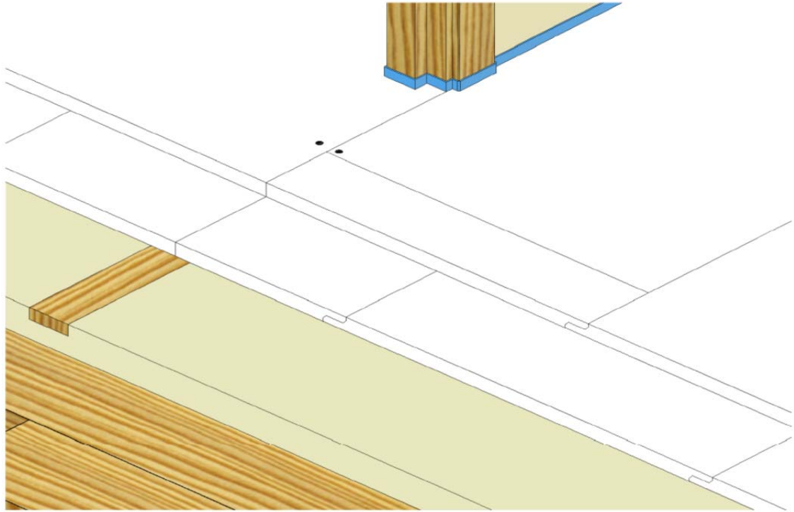
Figure 5 – KNAUF BRIO 18 double couche passage de porte
