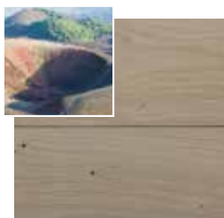
ETNA
