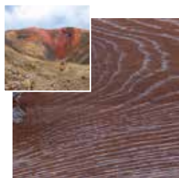
FUEGO
