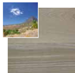
SOUFRIERE
