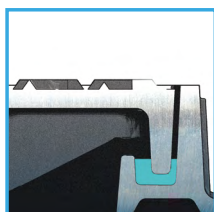
Gorge hydraulique > 6 mm : barrière aux remontées d'odeur
