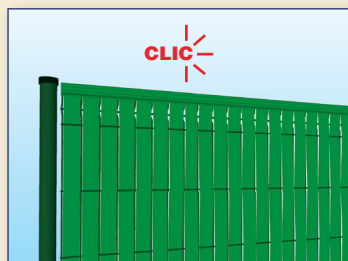
4. Verrouillez les LATTES avec la LISSE
