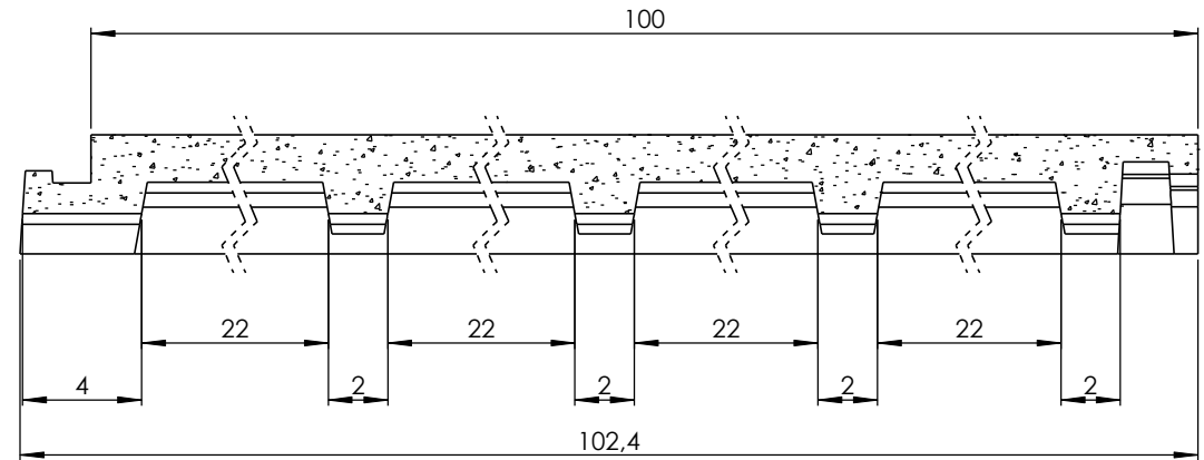
COUPE B-B
