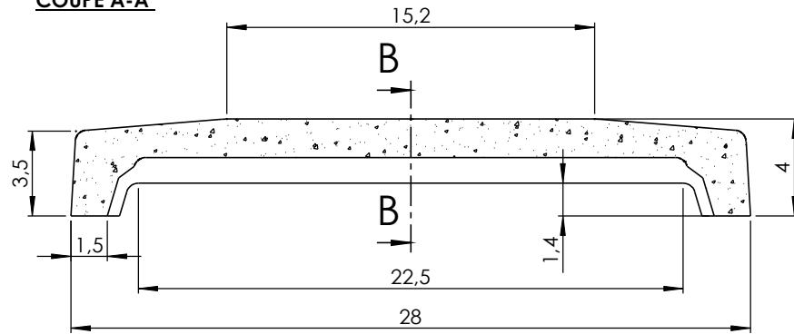
COUPE A-A
