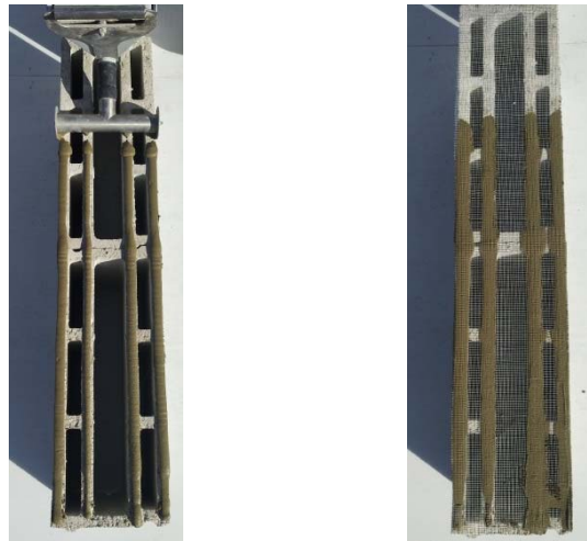
Figure 13 : Encollage de la trame tissée de verre
