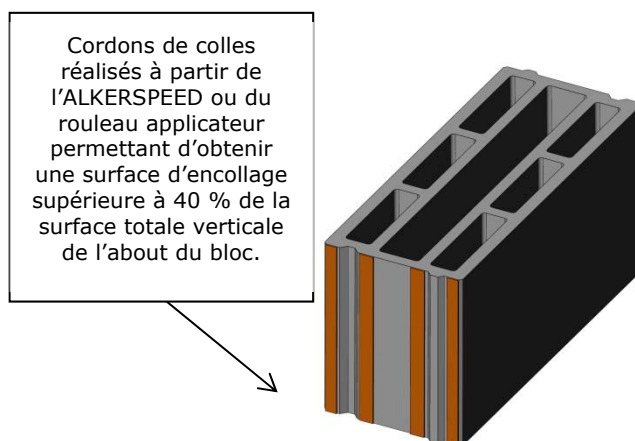
Figure 7 : Chants verticaux encollés
