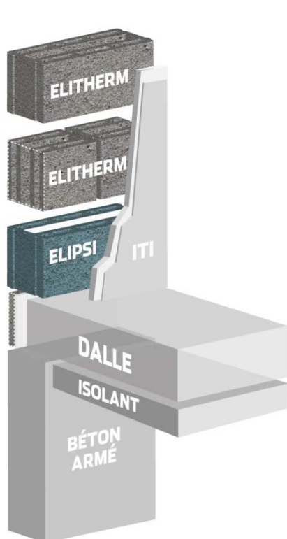
Exemple de traitement du pont thermique d'un plancher bas
