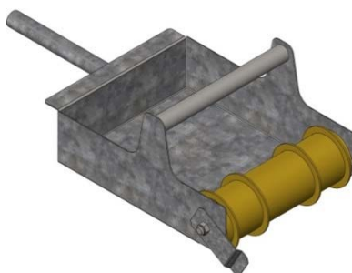
Figure 5 : Rouleau applicateur pour CONFORT R1, ELIPSI, ELITHERM
