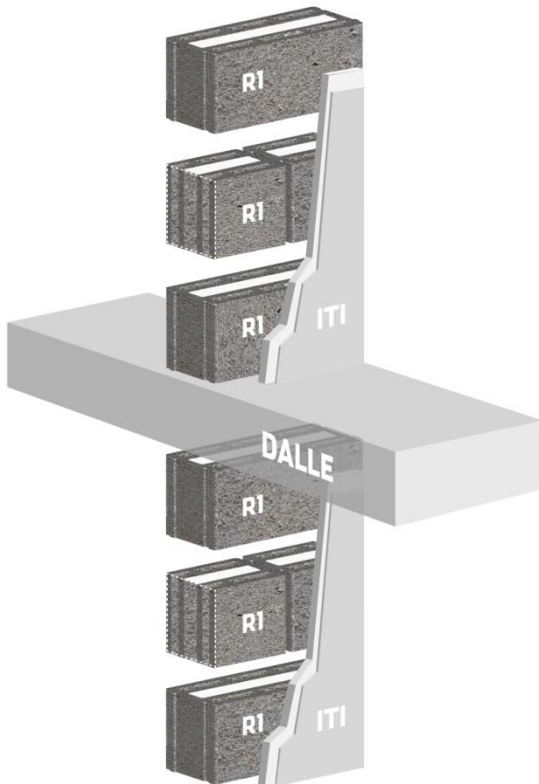
Exemple de traitement du pont thermique d'un plancher intermédiaire, au niveau d'un balcon
