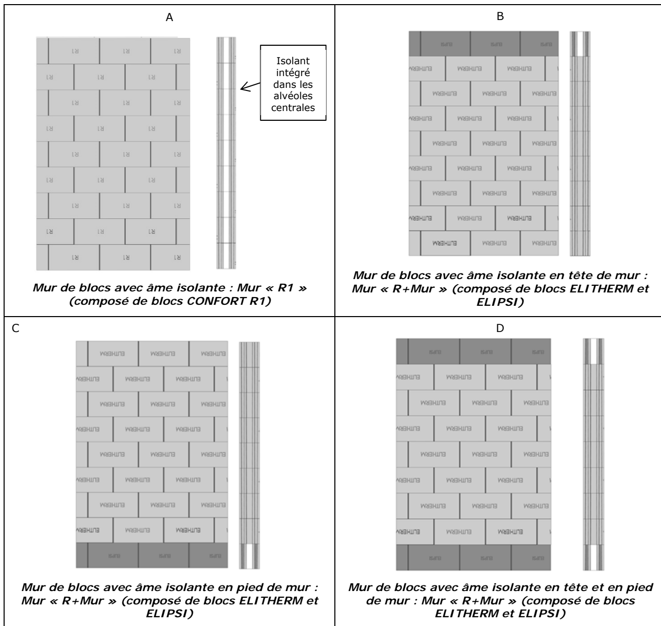
Figure 1 : Schémas de principes des différentes configurations envisageables
