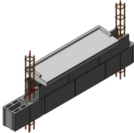
Figure 11 : Jonction par juxtaposition d'un mur de refend/mur de façade en zones non sismiques
