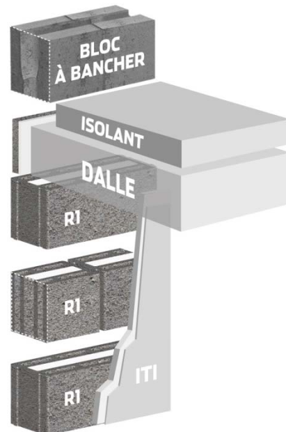
Exemple de traitement du pont thermique d'un plancher haut
