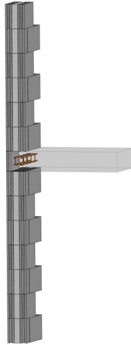
Figure 17 : Chaînage horizontal (appui de plancher) – Mur « R1 »
