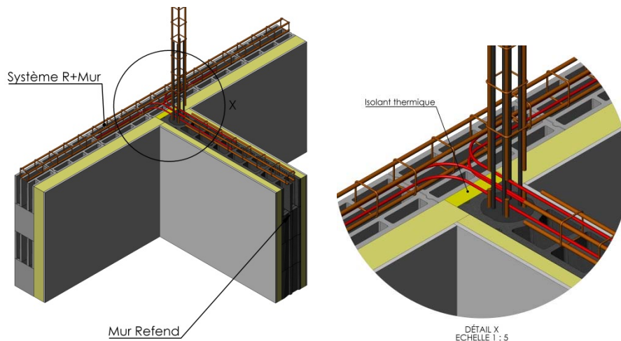
Figure 12 : Jonction par juxtaposition d'un mur de refend/mur de façade en zones sismiques
