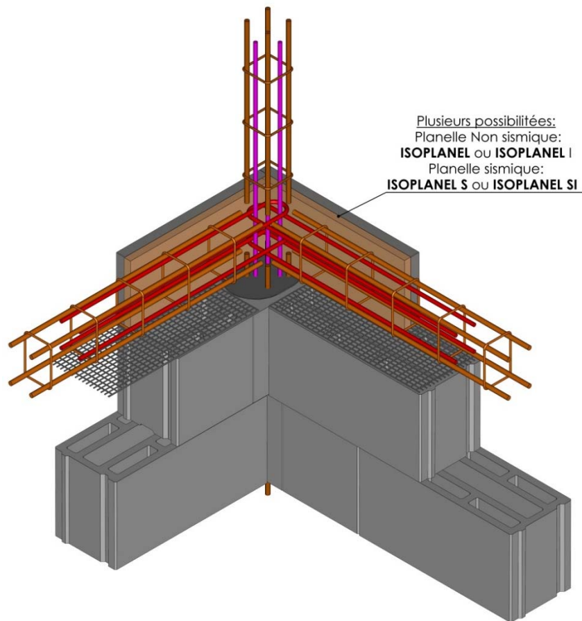
Figure 14 : Chainage horizontal (détail des armatures)
