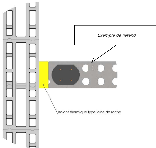
Figure 12 : Jonction par juxtaposition d'un mur de refend/mur de façade en zones sismiques
