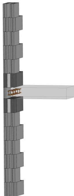
Figure 18 : Chaînage horizontal (appui de plancher) – Mur « R+Mur »
