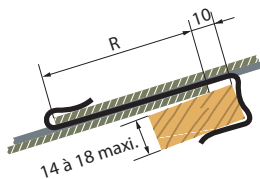
A - Crochet à pression pour lattage
