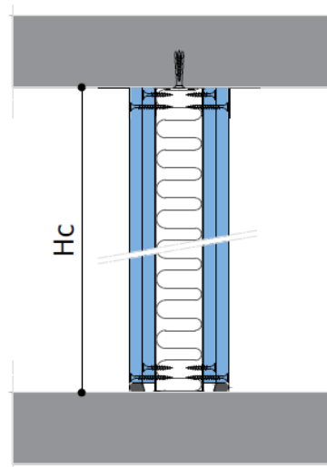
Coupe horizontale
