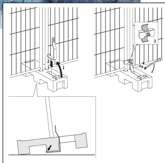
Systeme anti-levage pour plot sans eviderment E004045
