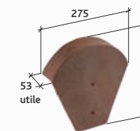
Fronton faitière 1/2 ronde Réf. 819
