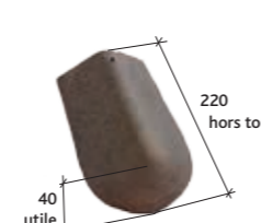
About d'arêtier Cornier Réf. 880
