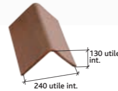
Faîtère angulaire sans emboîtement (3 au ml) Réf. 735
