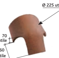
Rencontre 1 faîtère / 2 arêtiers Réf. 940
