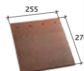
Tuile et demie 27 Réf. 520.95
