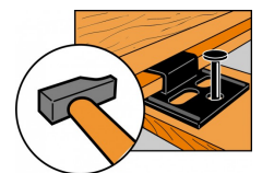
Fixation du CLIP par agrafe
