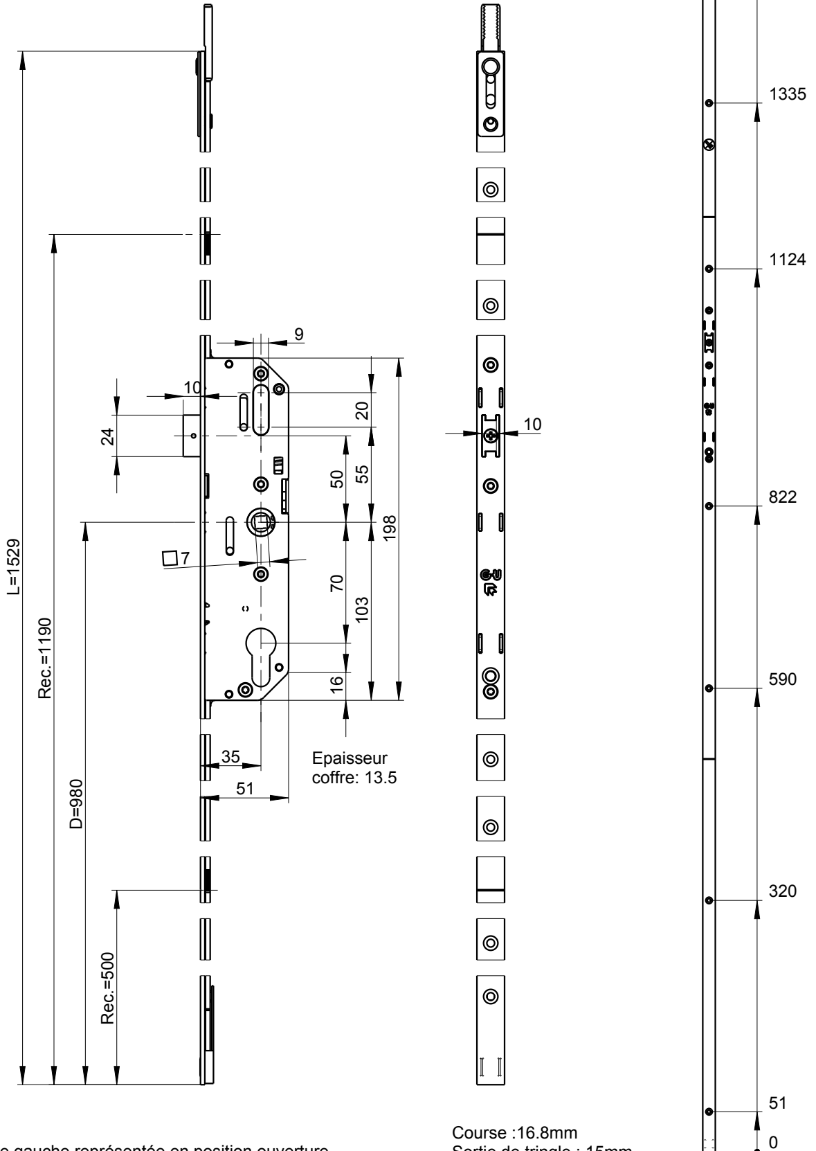
Crémone gauche représentée en position ouverture
