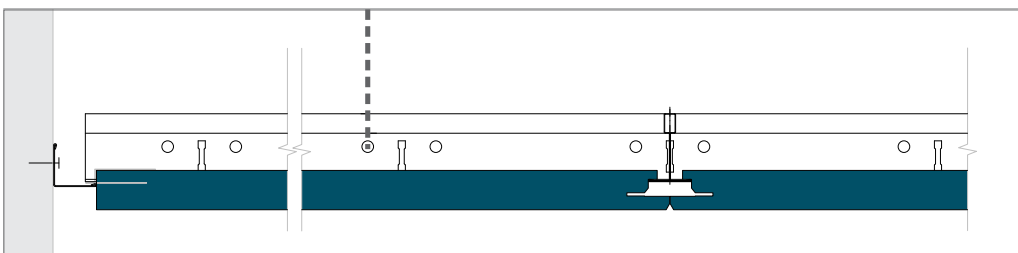
Finition périphérique avec clip mural pour créer un bord flottant.
