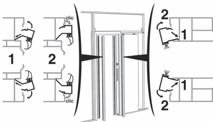
Clipsage / déclipsage des parcloses verticales
