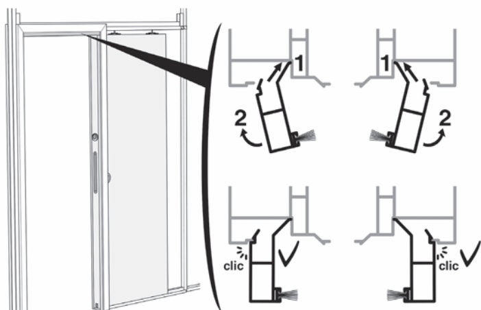
Clipsage / déclipsage de la parclose horizontale
