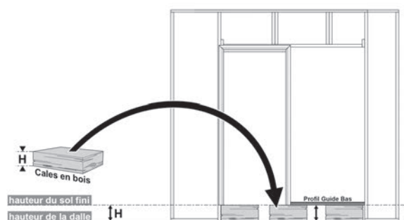
Schéma de pose de Navibloc® sur sol brut
