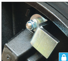
Kit de verrouillage RETROFIT disponible sur les SOLO D400 (544462 01)
