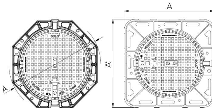
Kit de verrouillage RETROFIT disponible sur les SOLO D400 (544462 01)
