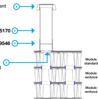
Module renforcé Wavin AquaCell Réf. 3087891
