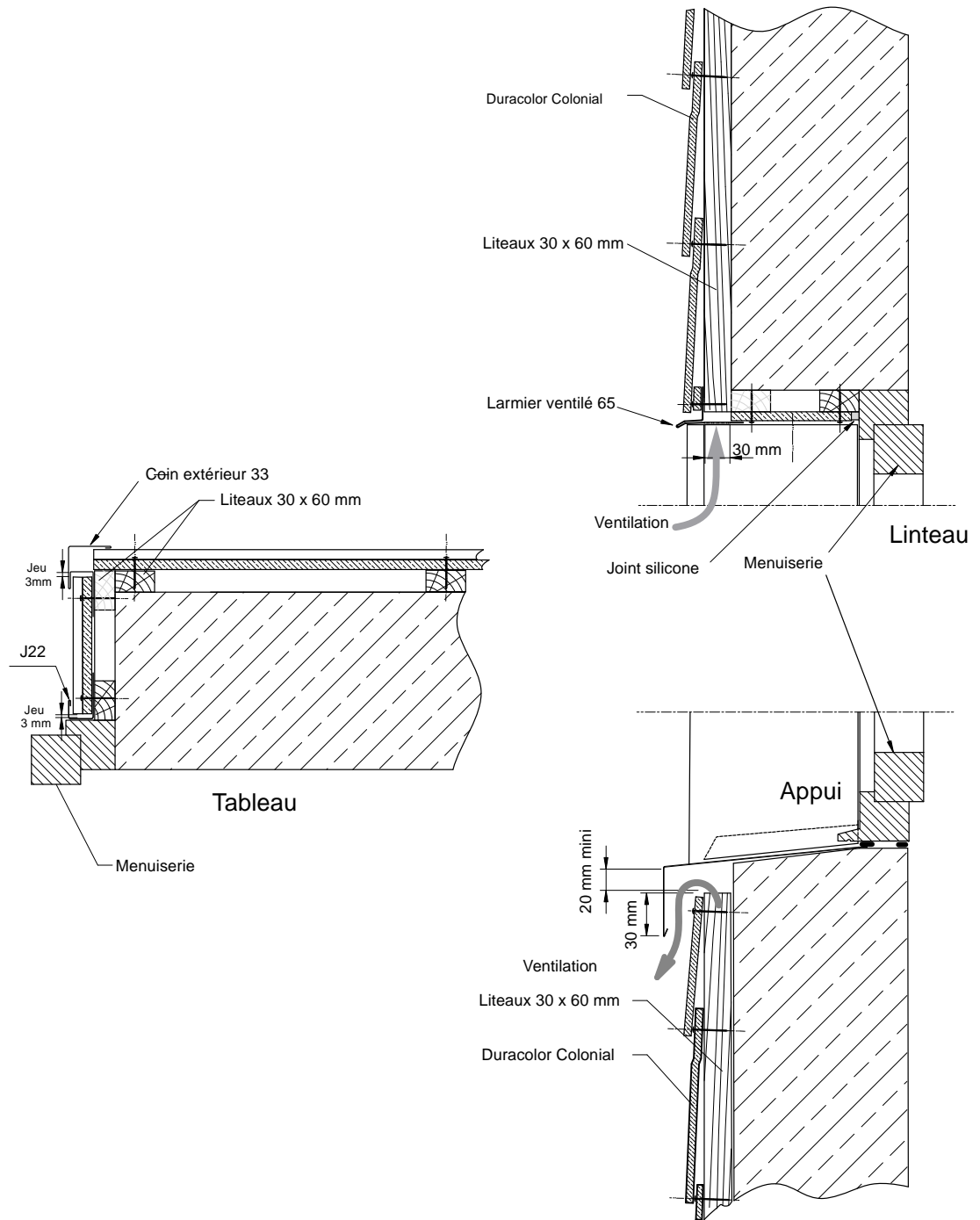
Figure 14 – Coupe sur menuiserie avec tableaux maçonnerie
