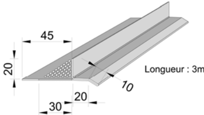
Larmier ventilé de 65
