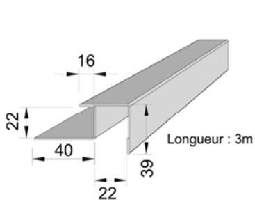
Coin extérieur continu 33
