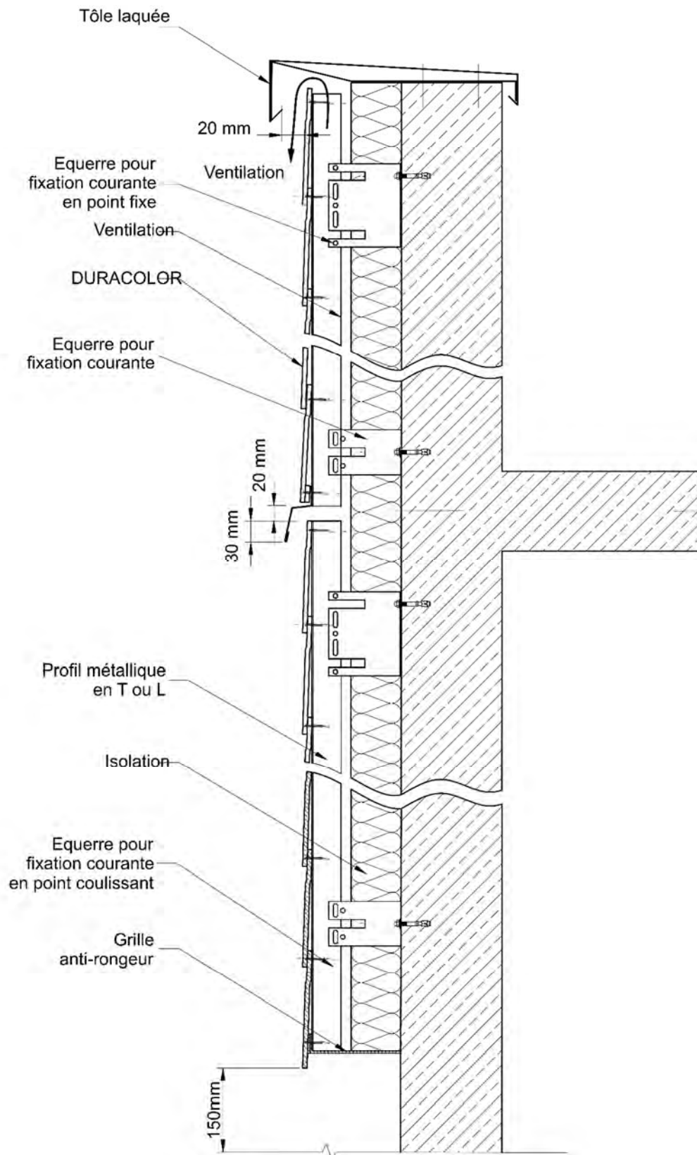
Figure 18 – Coupe sur bardage avec isolation ossature métallique sur gros-œuvre - fractionnement ossature et peau
