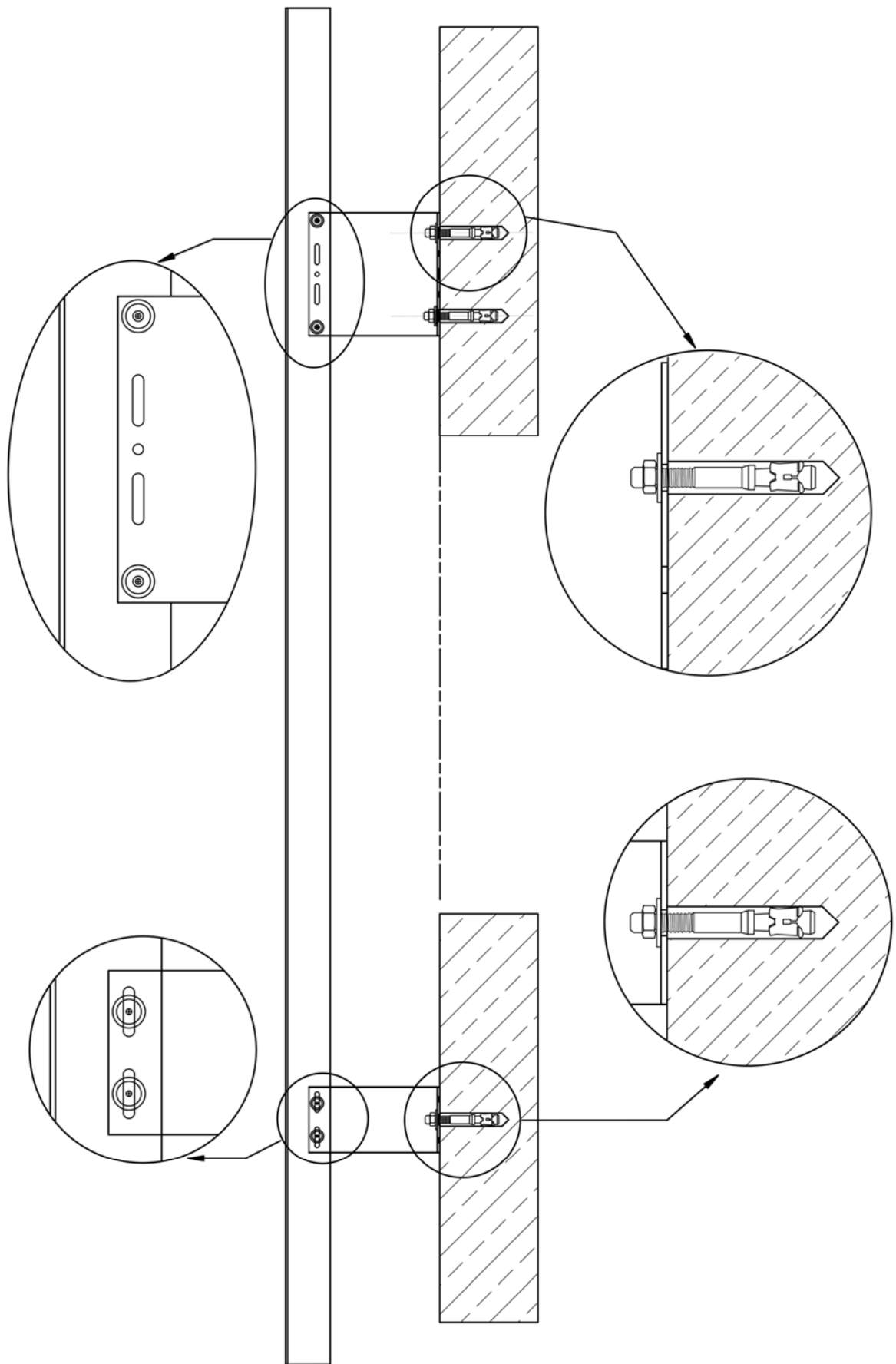
Figure B2 – Fixation des équerres sur le gros œuvre et positionnement - Fixation des profils sur pattes-équerres
