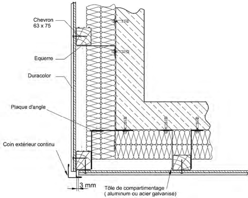
Angle sortant
