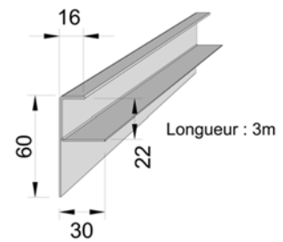
Moulure F22
