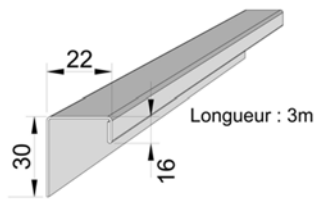
Moulure J22
