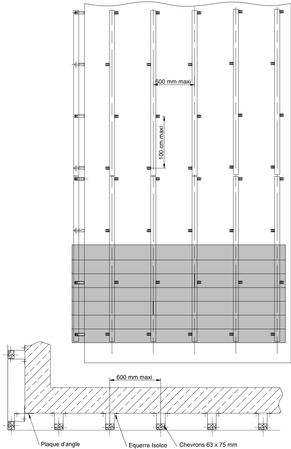
Figure A2 – Fixation des équerres – Ossature bois
