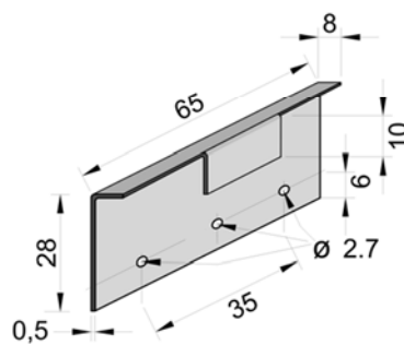
Clips fixation en inox pointes
