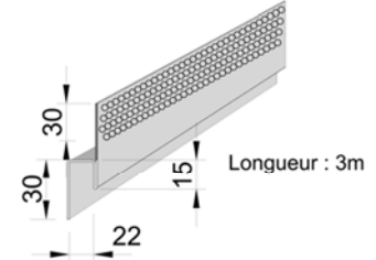
Grille de ventilation haute
