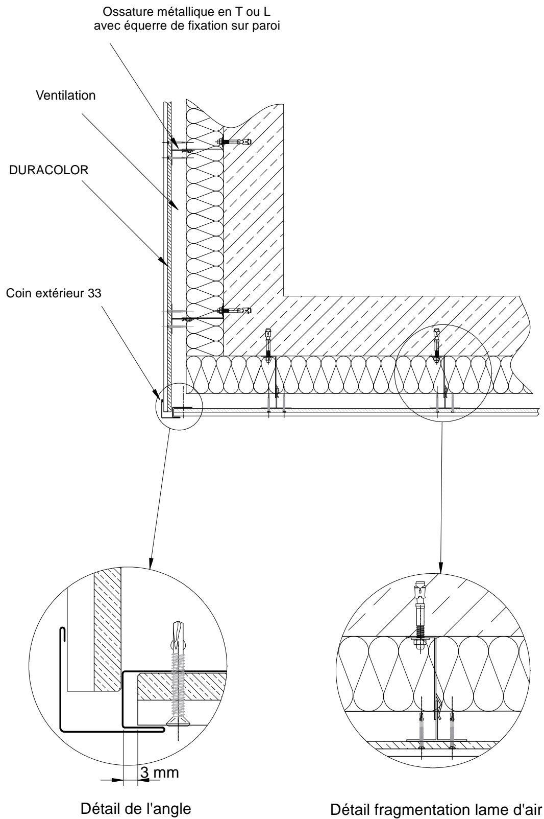
Figure 19 – Angle sortant – ossature métallique sur gros œuvre
