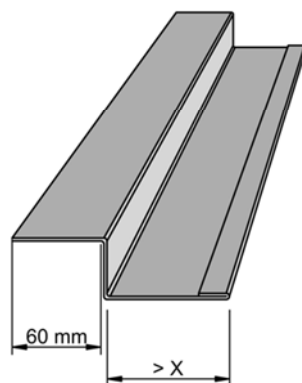
Figure 13 – Traitement de joint de dilatation longitudinal
