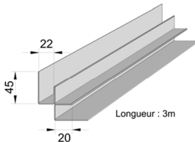
Coin intérieur continu
