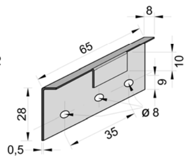
Clips fixation en inox Vis
