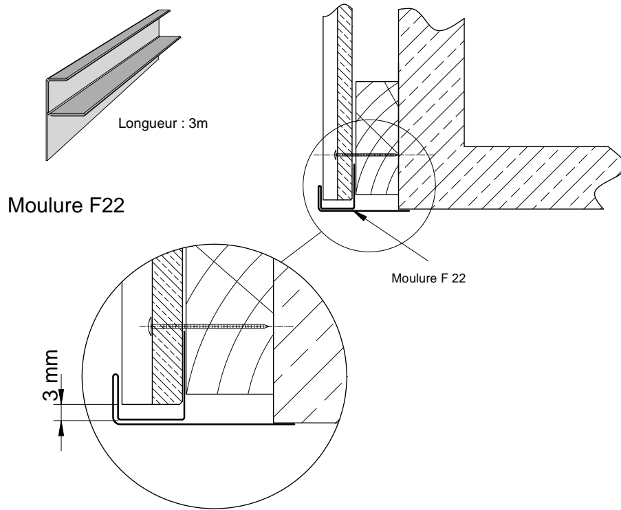
Figure 10 – Arrêt sur revêtement - Moulure F22 – Coupe horizontale
