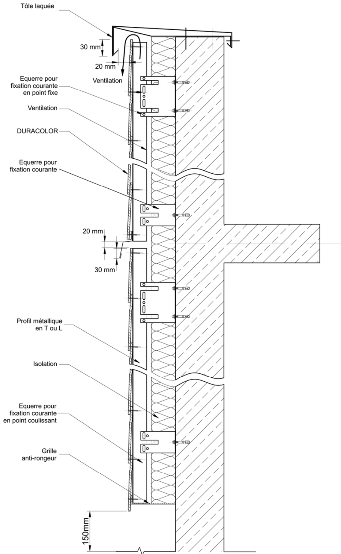
Figure B1 – Fractionnement de l'ossature métallique
