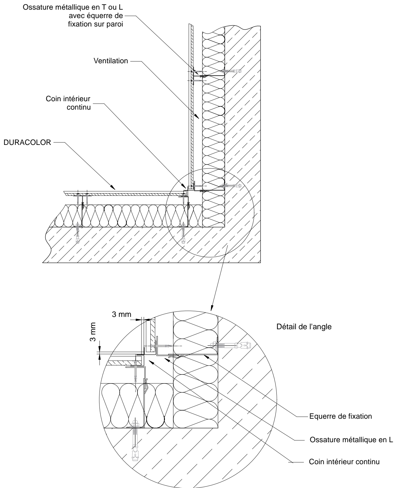
Figure 20 – Angle rentrant – Ossature métallique sur gros œuvre
