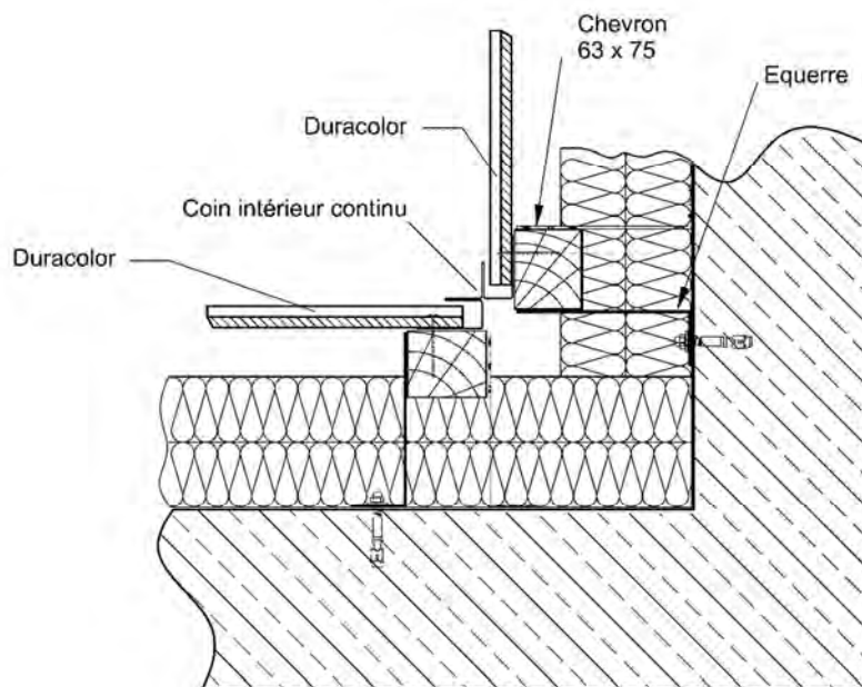
Angle rentrant
