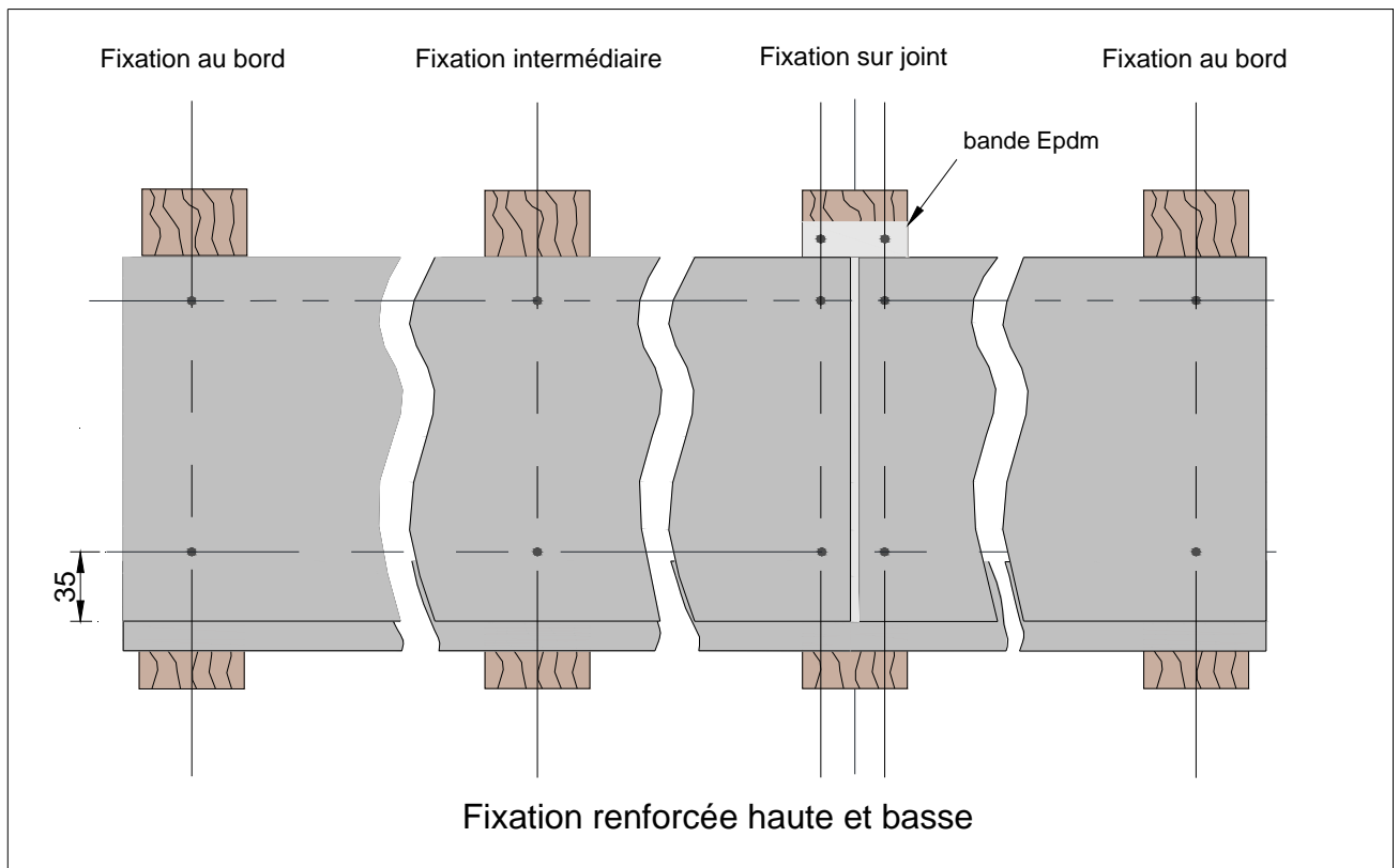
Figure 3.2 - Fixations des clips
