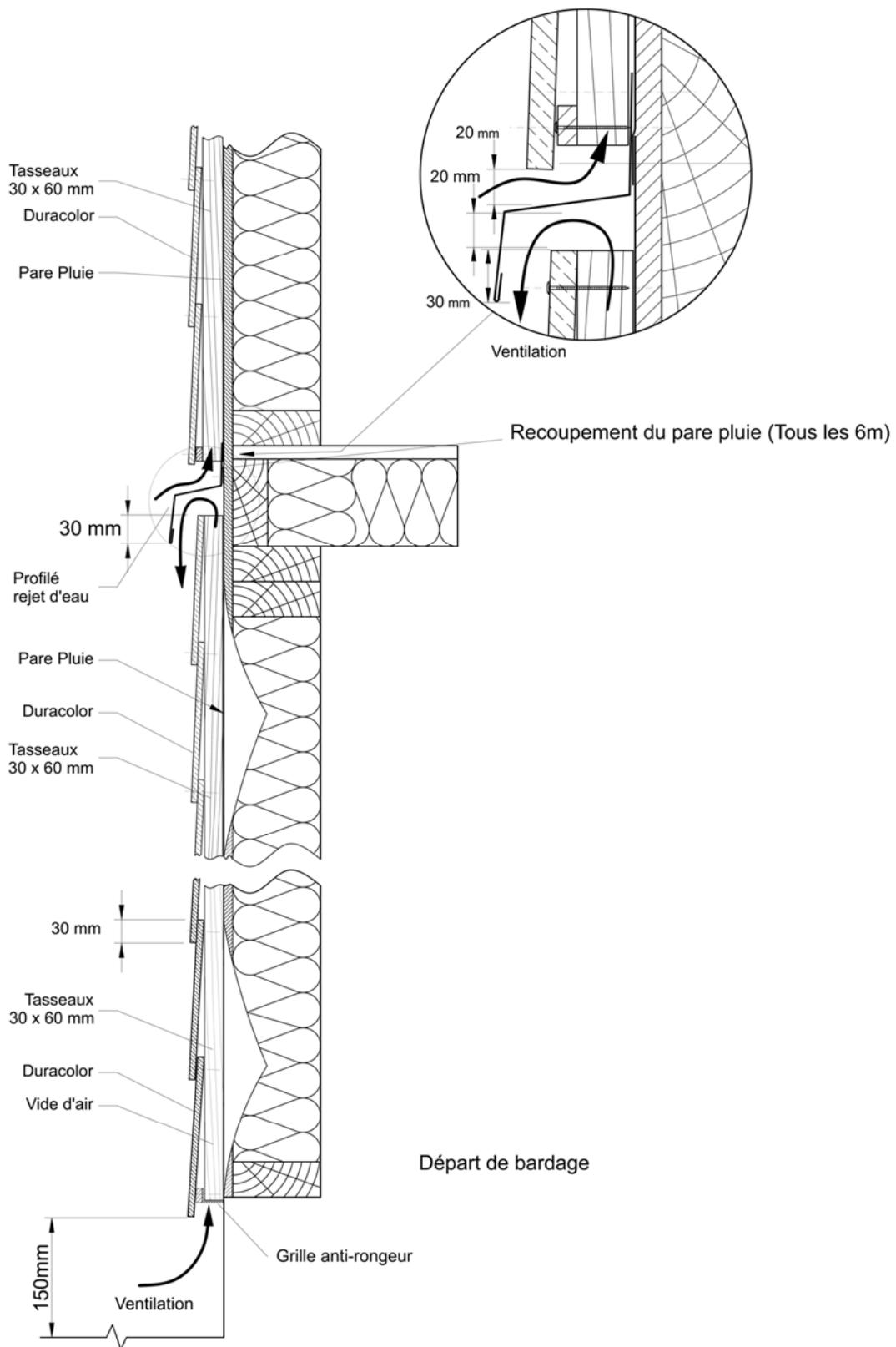
Figure 22 – Coupe verticale sur COB – Départ de bardage
