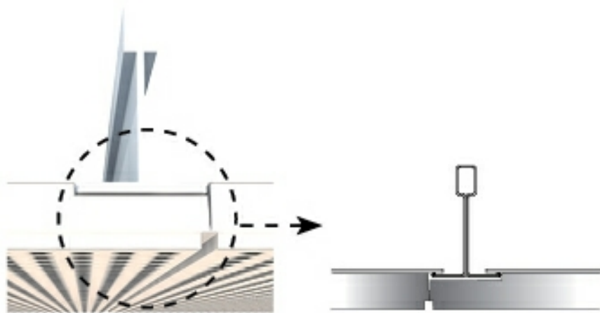
Nouveau Bord Contur D + avec ossature cachée démontable (T25)
