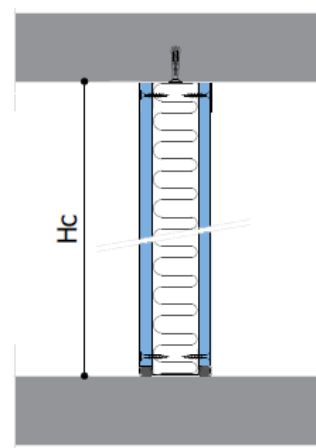
Coupe verticale
