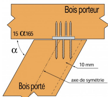
Assemblage en angle - Vue de dessus
