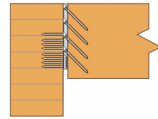
Fixation sur poutre (montage invisible avec lamage) Fixation sur poutre (montage apparent sans lamage)
